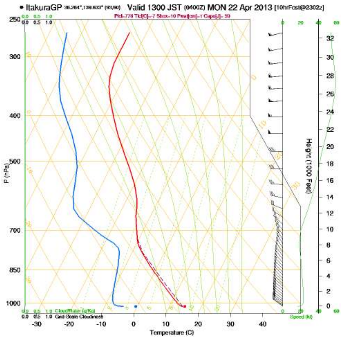
図9 板倉滑空場のエマグラムの例
